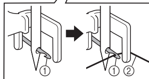
1 Гачок 2 Нитка • Тримайте нитку перед голкою, щоб переконатися, що гачок її схопить.
