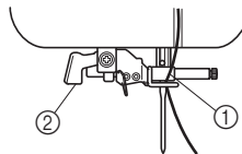
1 Тримач голки 2 Важіль інструмента для вставлення нитки в голку
