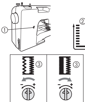
① Гвинт точного регулювання петлі ② Ліва сторона ③ Зовнішній вигляд петлі
